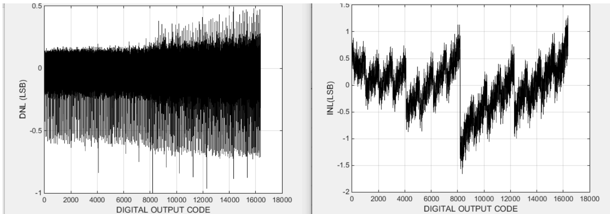
图 6-1 DNL 与 INL
