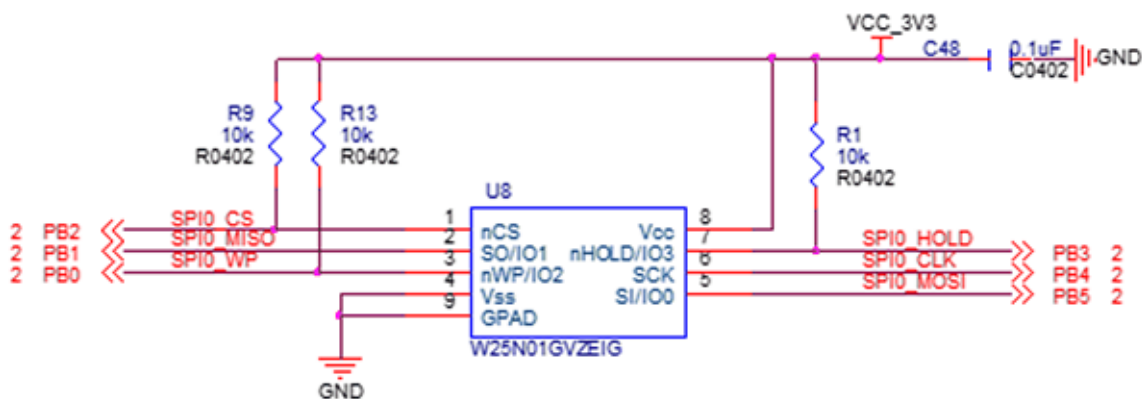
图 2-3 SPI0 NAND Flash 电路原理图
