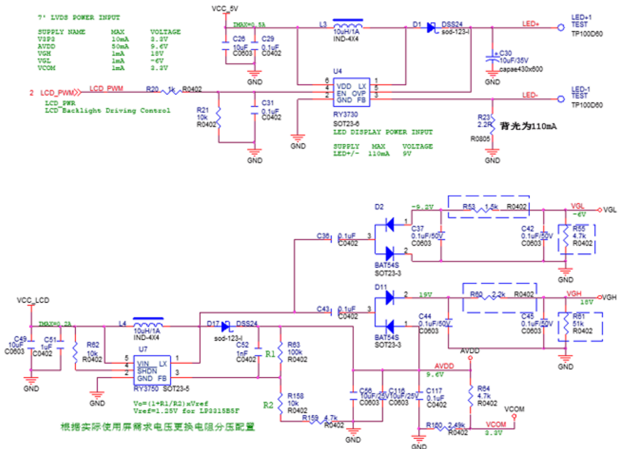
图 2-16 LCD 背光和偏压电路原理图
