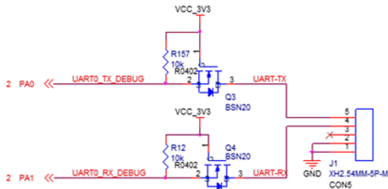
图 2-26 串口调试打印电路原理图
