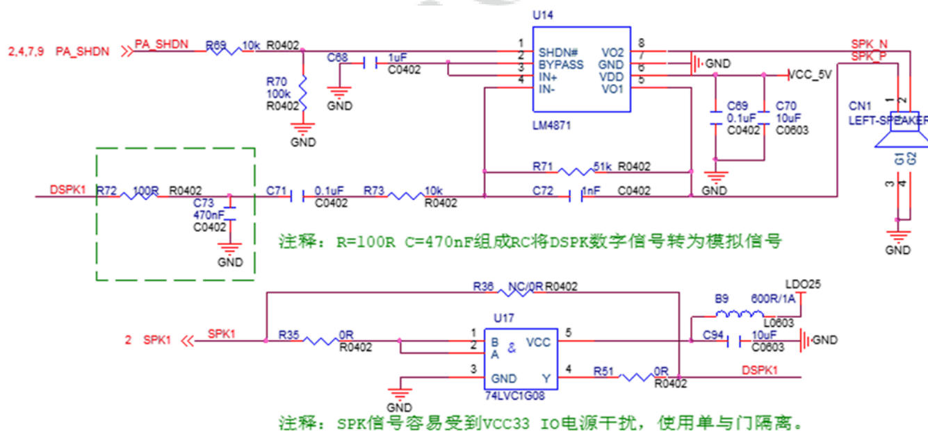
图 2-21 Speaker 单端输出电路原理图
