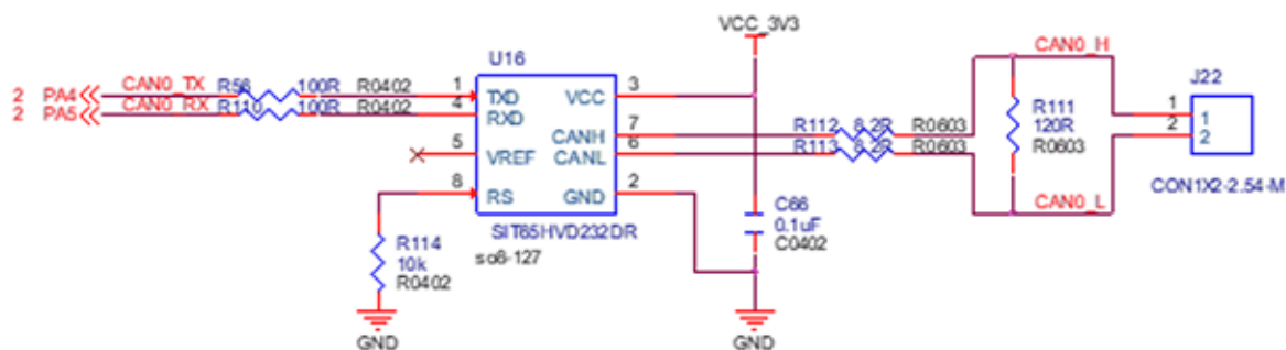
图 2-31 CAN 电路原理图
