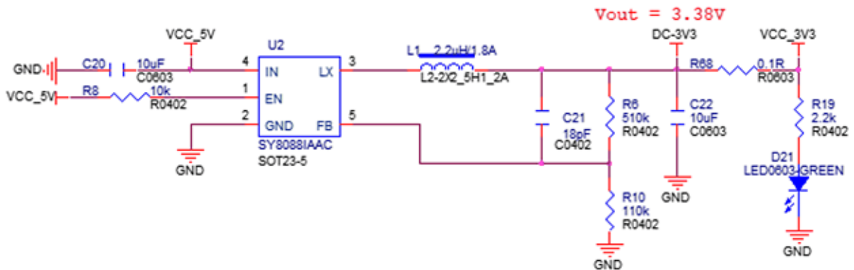
图 2-2 芯片 IO 电源 VCC33_IO 原理图
