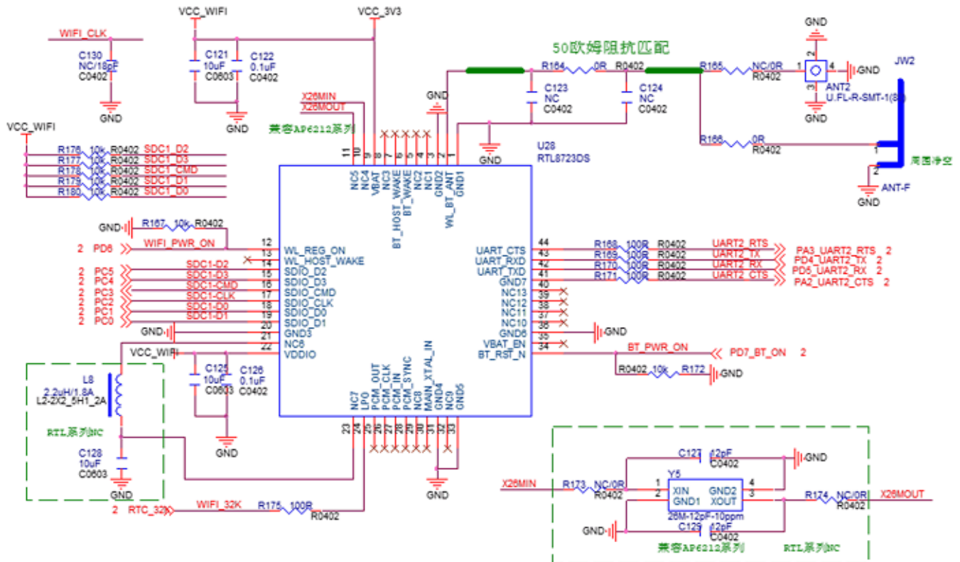
图 2-36 SDC1 WiFi+BT 电路原理图
