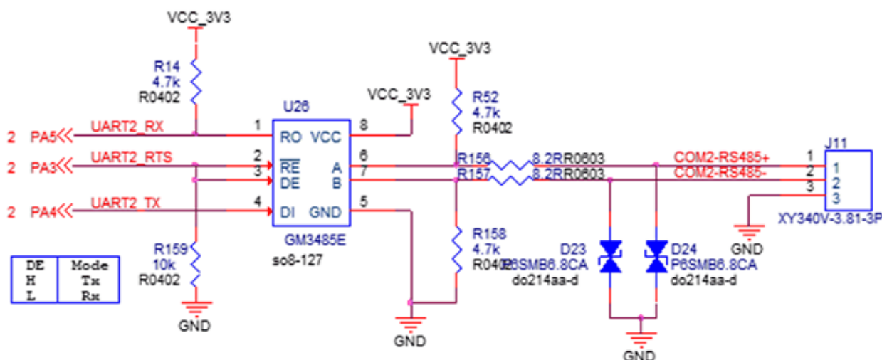
图 2-29 RS485 三线接法电路原理图
