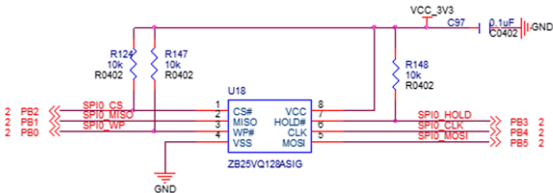
图 2-4 SPI0 NOR Flash 电路原理图
