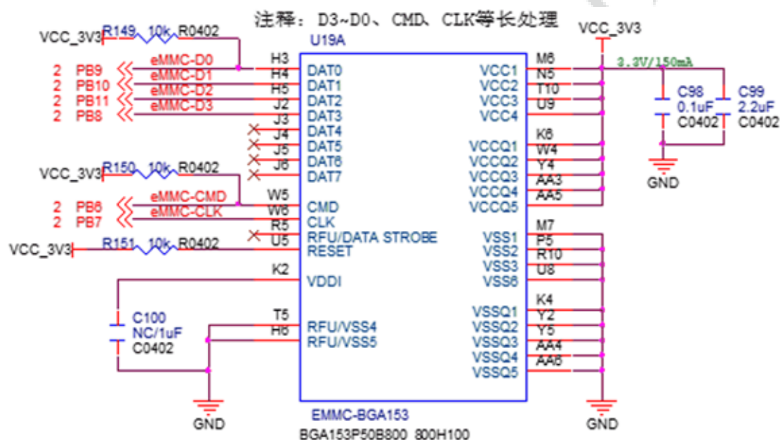
图 2-5 SDC0 eMMC 电路原理图
