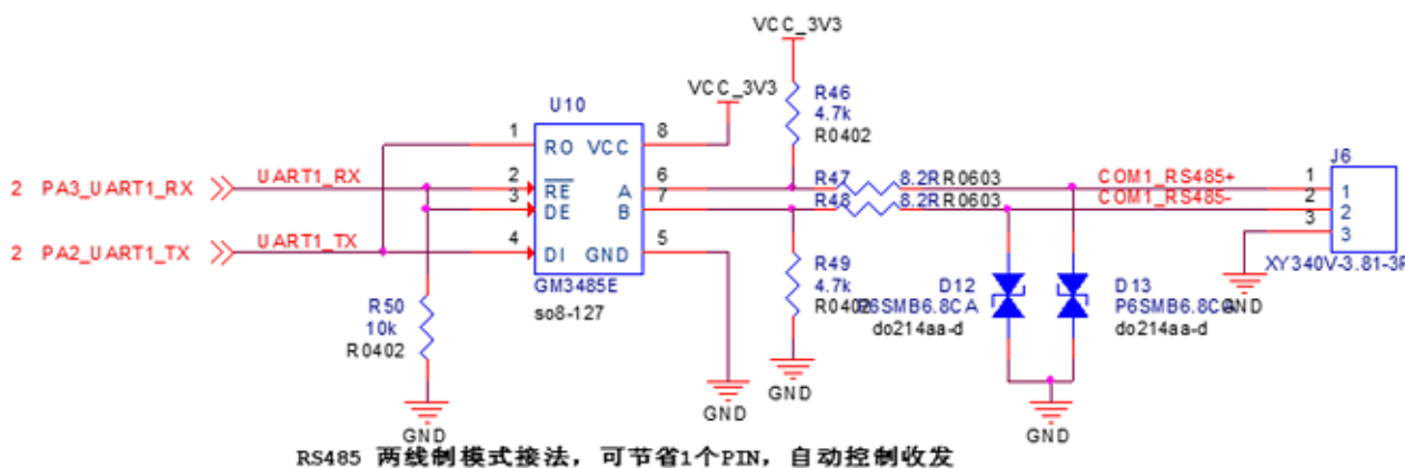
图 2-28 RS485 两线接法电路原理图
