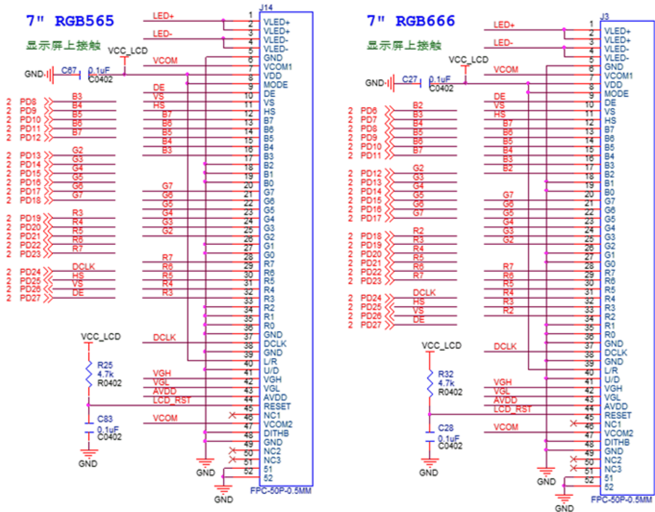
图 2-8 RGB565 / RGB666 电路原理图
