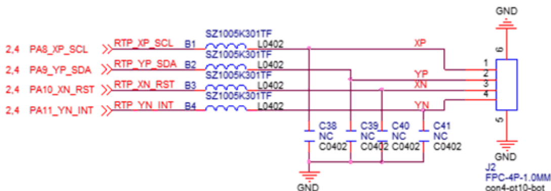
图 2-14 RTP 电阻屏触摸电路原理图
