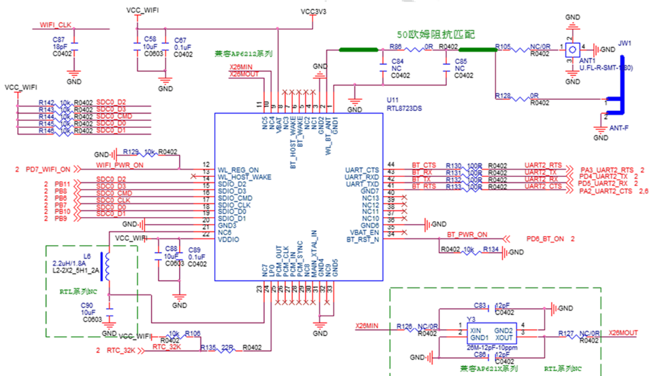
图 2-35 SDC0 WiFi+BT 电路原理图
