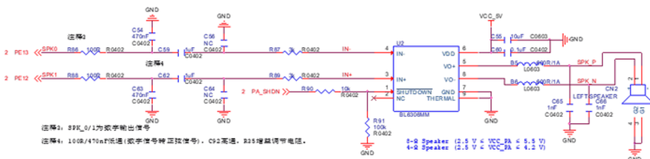
图 2-20 Speaker 差分输出电路原理图
