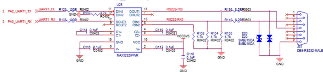
图 2-27 RS232 串口电路原理图
