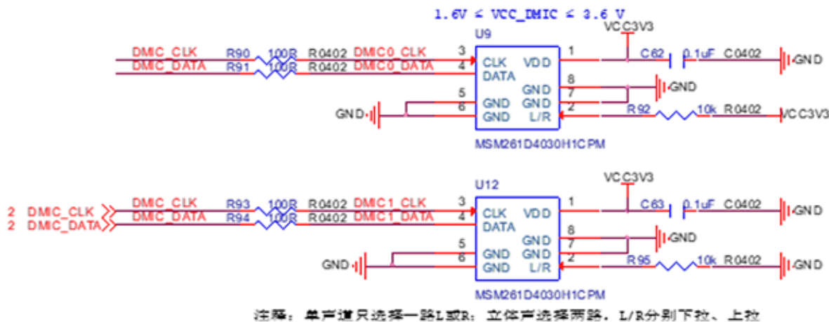
图 2-19 DMIC 电路原理图
