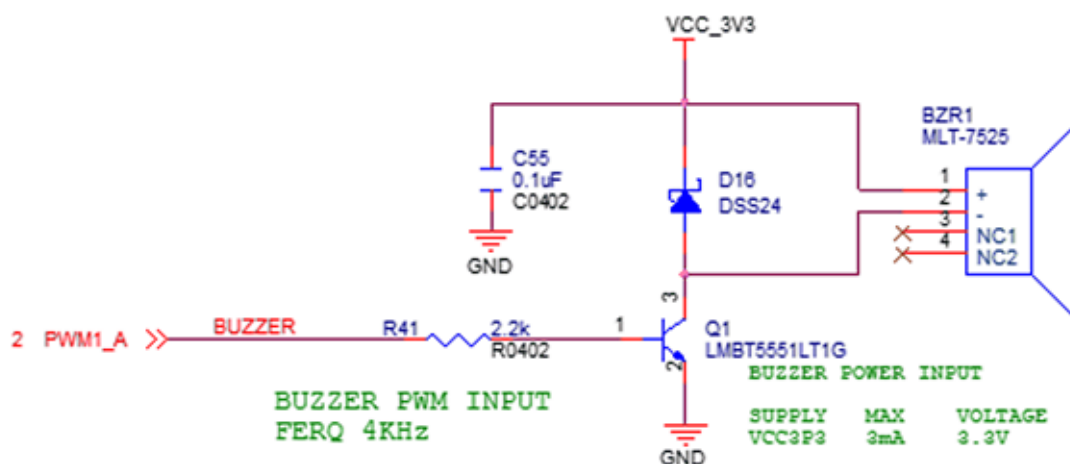
图 2-17 蜂鸣器电路原理图
