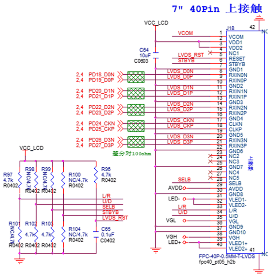
图 2-10 LVDS Single-Link 电路原理图
