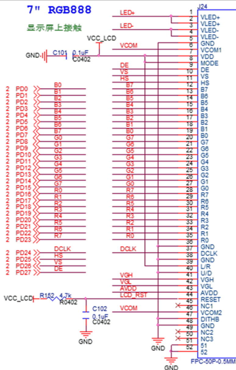
图 2-9 RGB888 电路原理图
