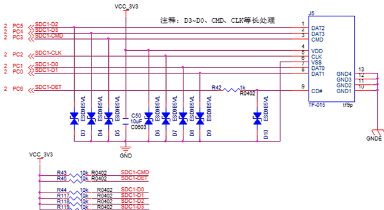
图 2-6 SDC1 CARD 电路原理图
