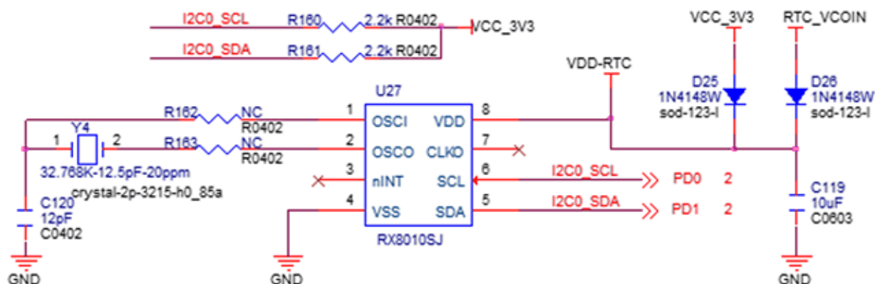
图 2-30 I2C 外接 RTC 电路原理图
