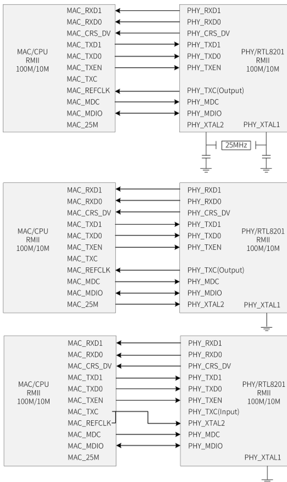
图 2-23 RTL8201 三种接法框图
