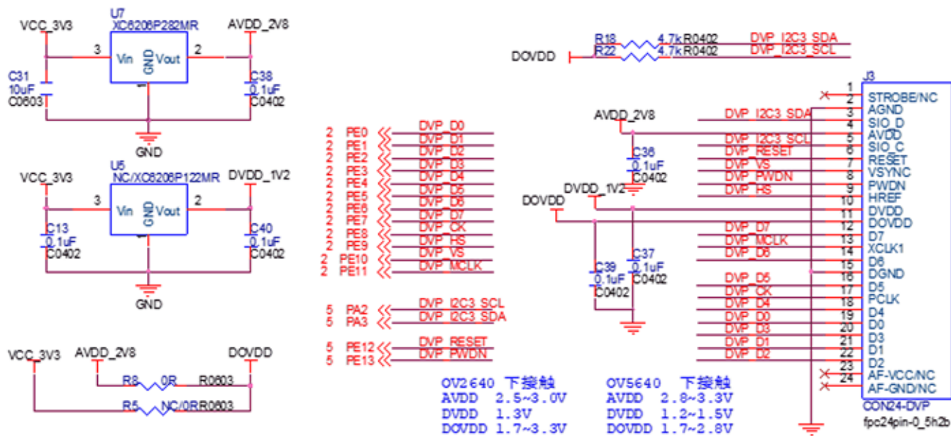
图 2-18 DVP CAMERA 原理图
