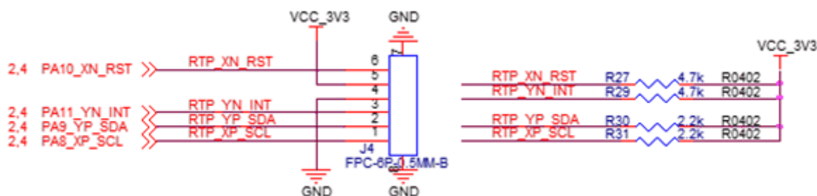
图 2-15 CTP 电容屏触摸电路原理图
