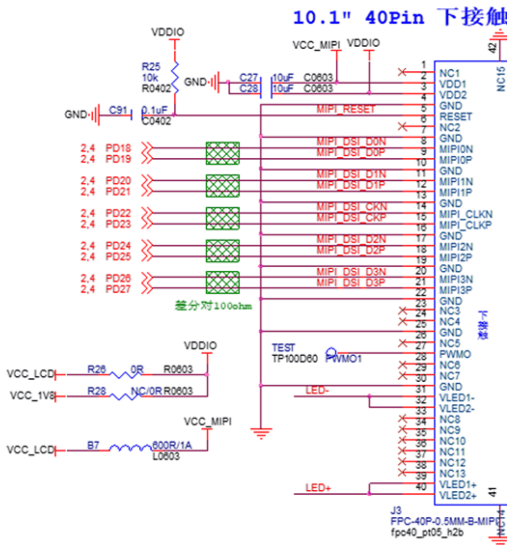
图 2-11 MIPI-DSI 电路原理图
