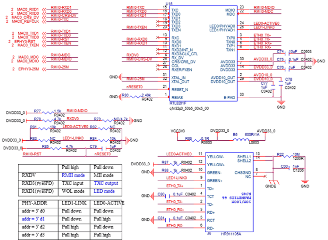
图 2-25 RTL8201 RMI 电路原理图
