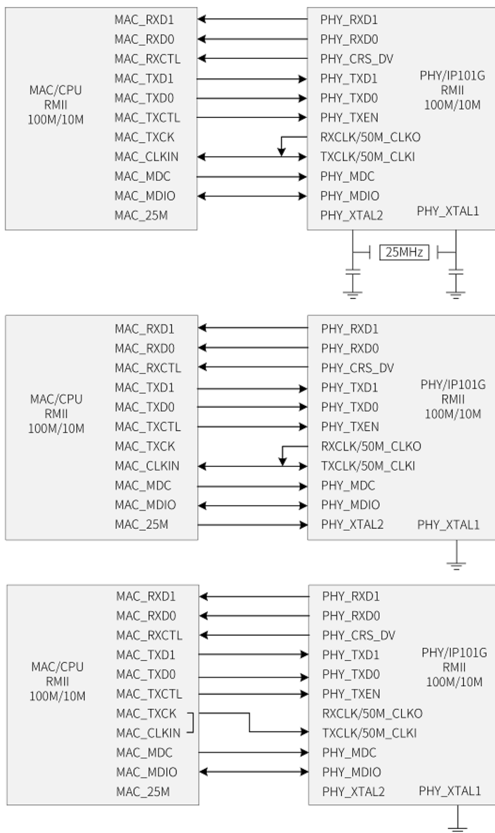
图 2-24 IP101G 三种接法框图
