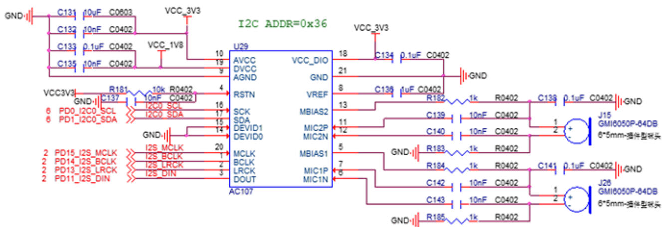
图 2-22 I2S 扩展麦克风电路原理图
